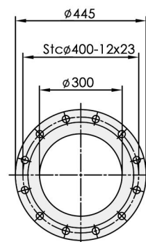
ZUIG-/PERSFLENS VOLGENS EN1092-2 DN300 PN10
