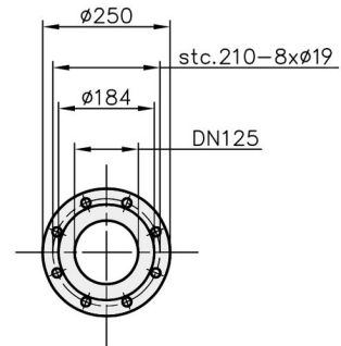
ZUIG- EN PERS FLENS DN125 EN1092-2 PN16 (GELIJK AAN PN10)
