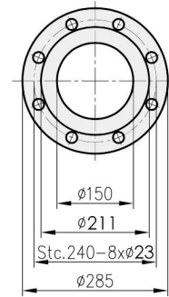
FLENS PN10 & PN16 (GELIJK) VOLGENS NORM EN1092-2
