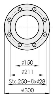
FLENS PN25 VOLGENS NORM EN1092-2
