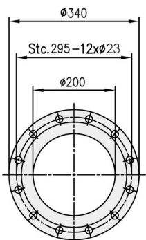
FLENS PN16 VOLGENS EN1092-2 DN200
