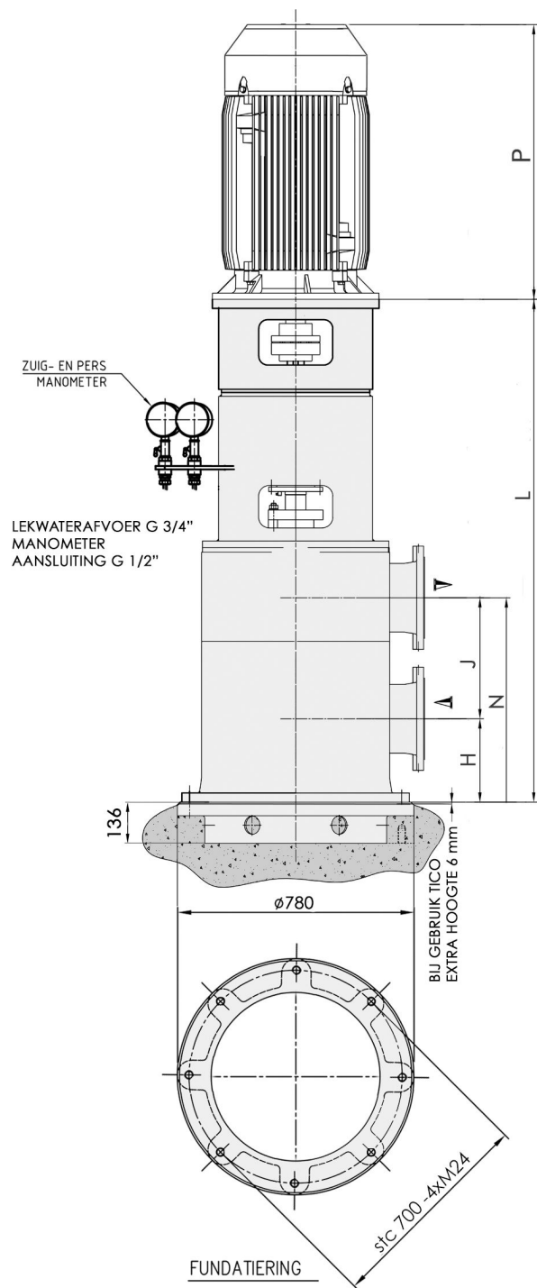
FLENS PN10 VOLGENS EN1092-2 DN200
