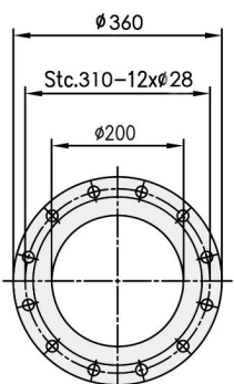
FLENS PN25 VOLGENS EN1092-2 DN200
