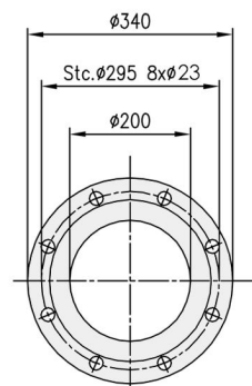
FLENS PN10 VOLGENS EN1092-2 DN200
