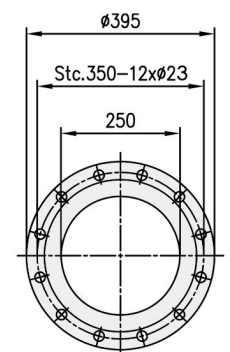
ZUIG-/ PERSFLENS VOLGENS EN1092-2 DN250 PN10
