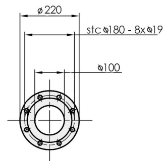
ZUIG- EN PERS FLENS DN100 EN1092-2 PN16 (GELIJK AAN PN10)
